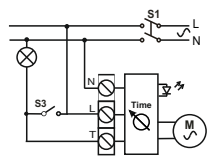
Схема электрическая 4
